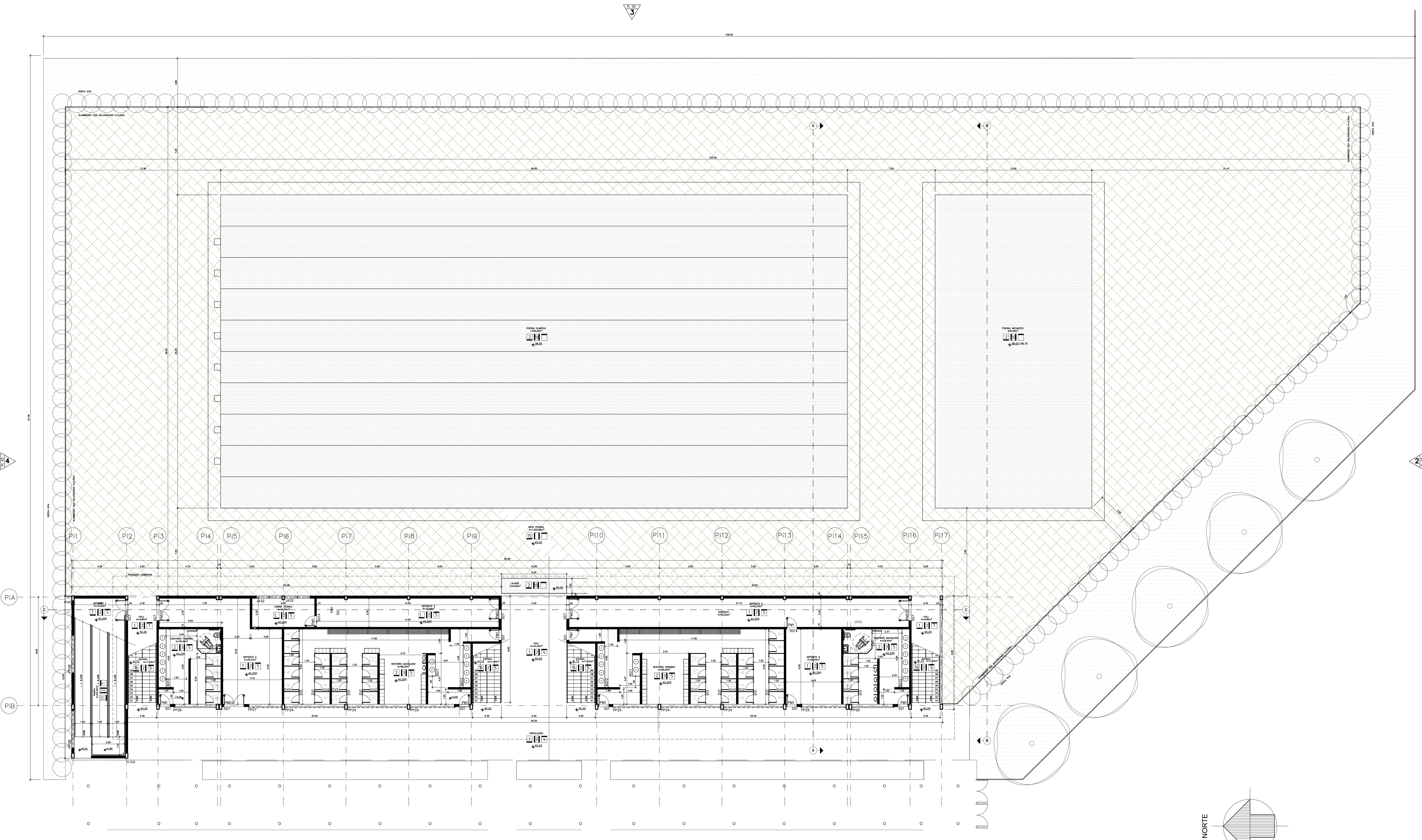
PLANTA TERREO/IMPLANTAÇÃO escala 1:100
