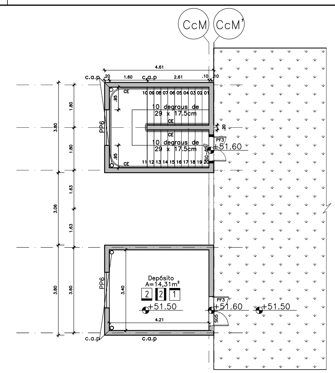
PLANTA NÍVEL 51.50—ACESSO A COBERTURA VERDE esc. 1/100
